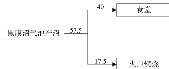
图 2.4-2 沼气平衡图 (单位: \text{m}^3/\text{d} )
