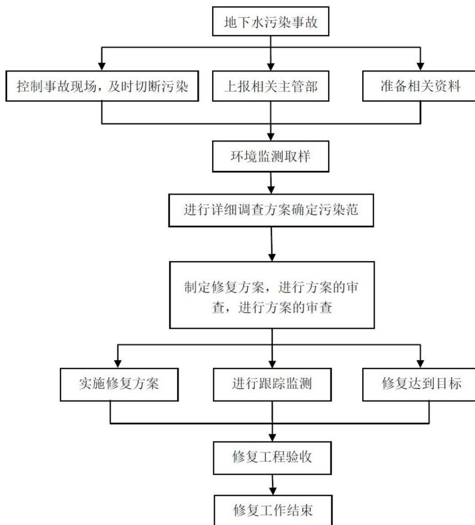
图 7.2-3 地下水污染应急治理程序框图
