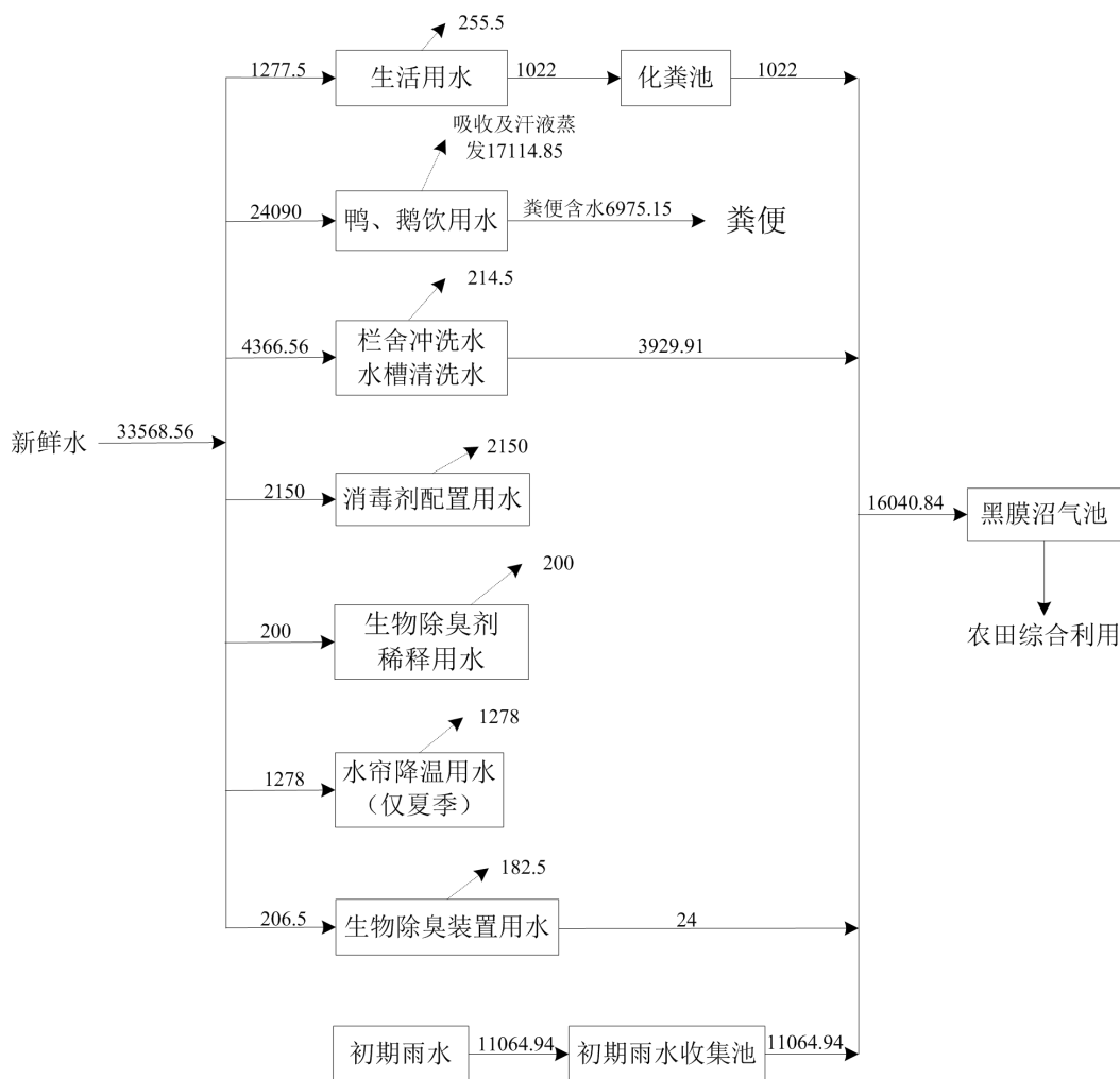
图 2.4-1 项目水平衡图 (单位: m³/a)
