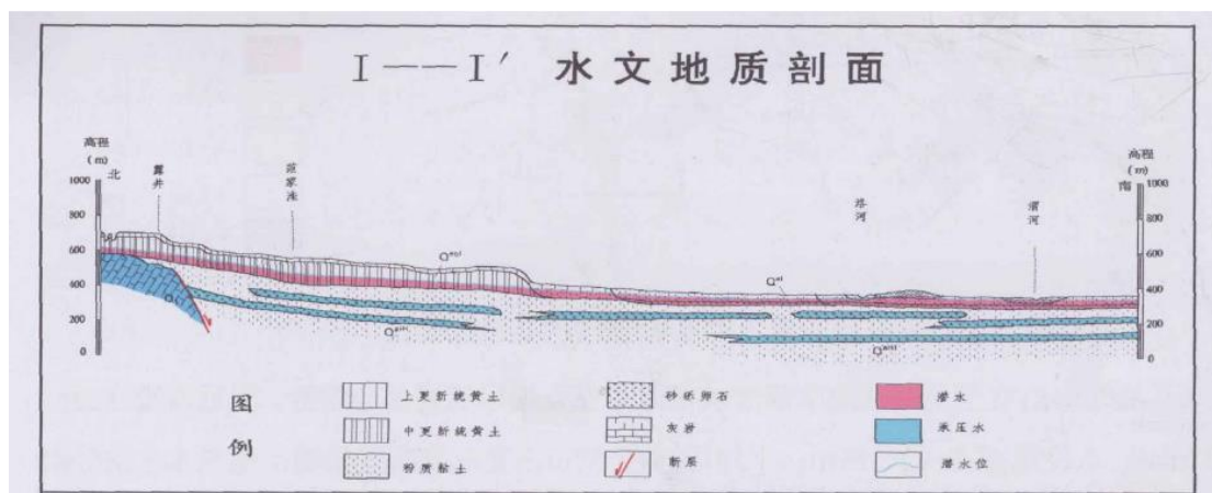
图 5.2-3 大荔县潜水水文地质剖面图
