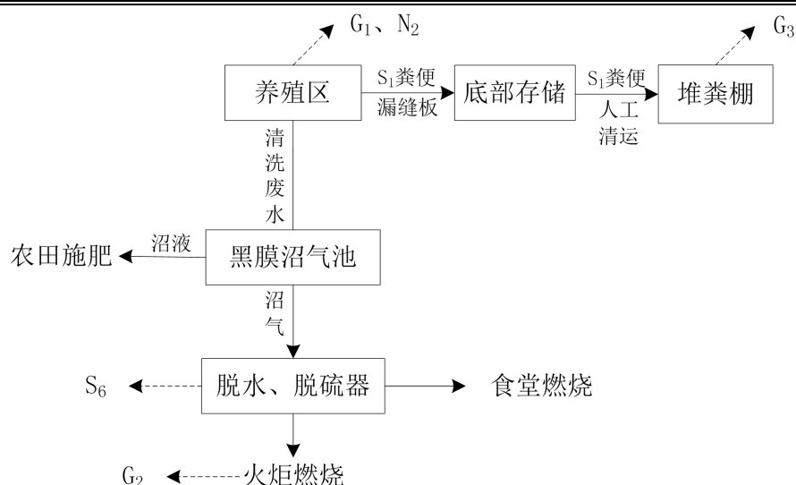
图 7.2-1 养殖废水处理工艺流程图
