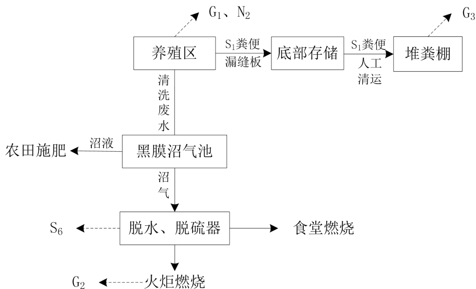
图 2.3-3 粪污水处理工艺流程及产污环节图
