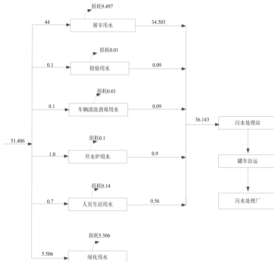
图 2-1 项目水平衡图 (m³/d)
